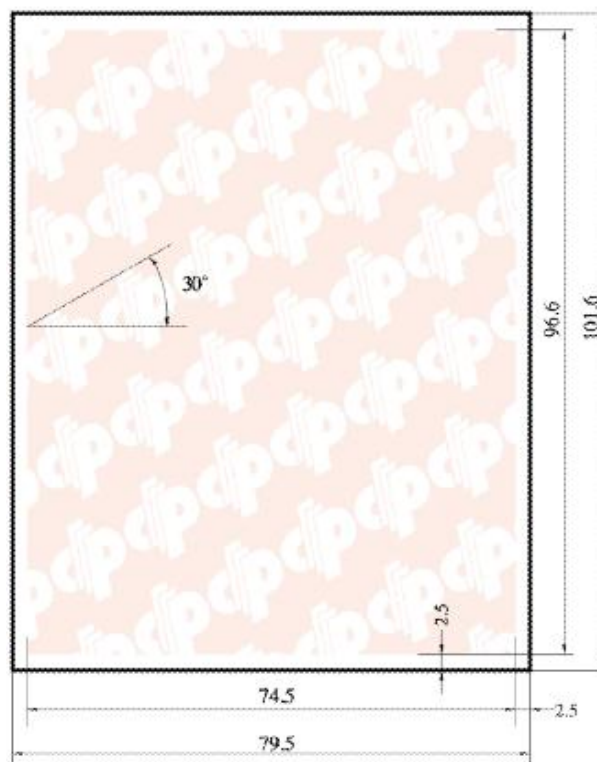
图 2 底纹区域图案示意图 单位: mm
